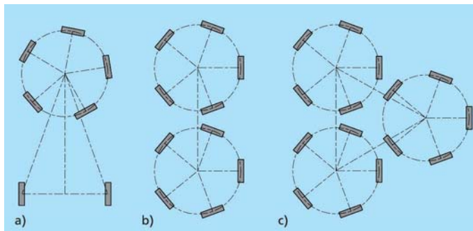
4 Mögliche Ausführungen der Fahrwerke
